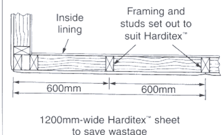
Fig. 11 FRAME AND STUD SET-OUT
